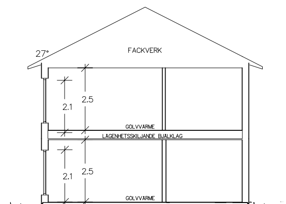
SEKTION A-A
